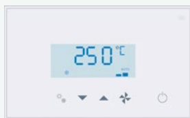
Controlador de sala táctil Modbus RS-485 con E/S, blanco.
