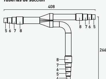
Tuberías de succión
