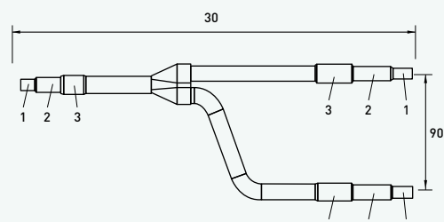
Tubería de líquido
