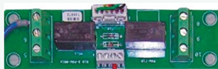
PCB de interfaz T10 con conexiones digitales y de relé.
