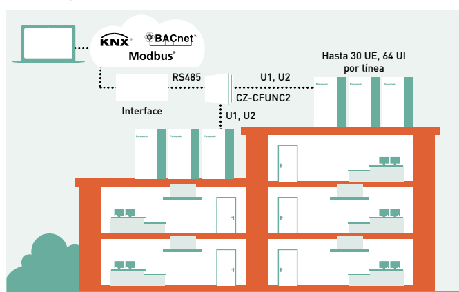
Interfaz antigua.
